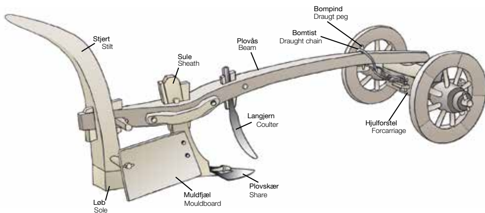
Fig. 1. Rekonstruktion af muldfjælspløven på baggrund af genstandsfund samt paralleler til tilsvarende plove i museernes samlinger, der i hovedsagen tilhører den sidste periode af pløjeredskabets historie fra ca. 1750-1850. – Tegning: Jørgen Andersen, Museum Sønderjylland efter Lerche 1994.
